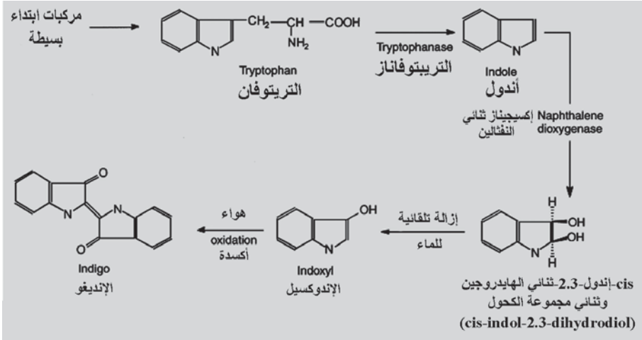
الشكل 2.24 مسار أيض وهندسة تخليق الإنديغو (Indigo Biosynthesis).
